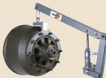
Hubvorrichtung HV 3 mit ECO-Bremstrommel von BPW.
